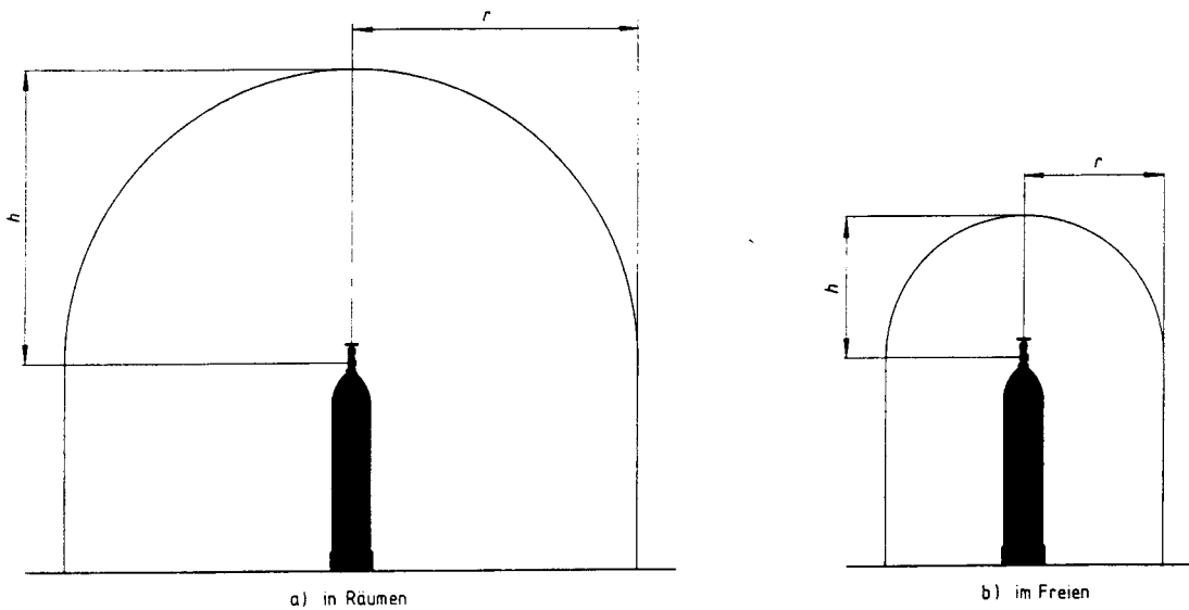
Bild 1 Schutzbereiche für Druckgasflaschen mit Gasen, die leichter als Luft sind
