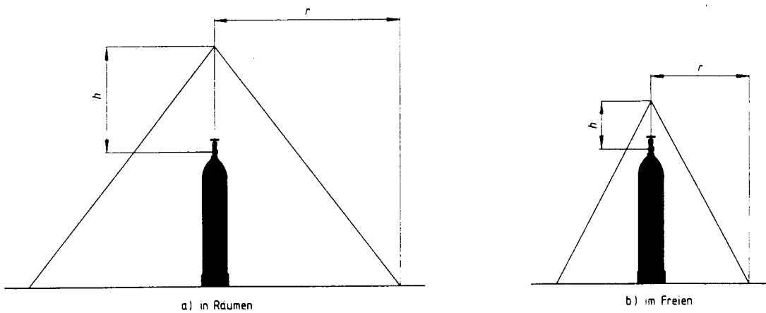
Bild 2 Schutzbereiche für Druckgasflaschen mit Gasen, die schwerer als Luft sind
